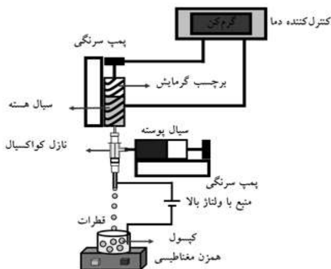
شکل ۳- الکترورسی مواد تغییر فازدهنده
