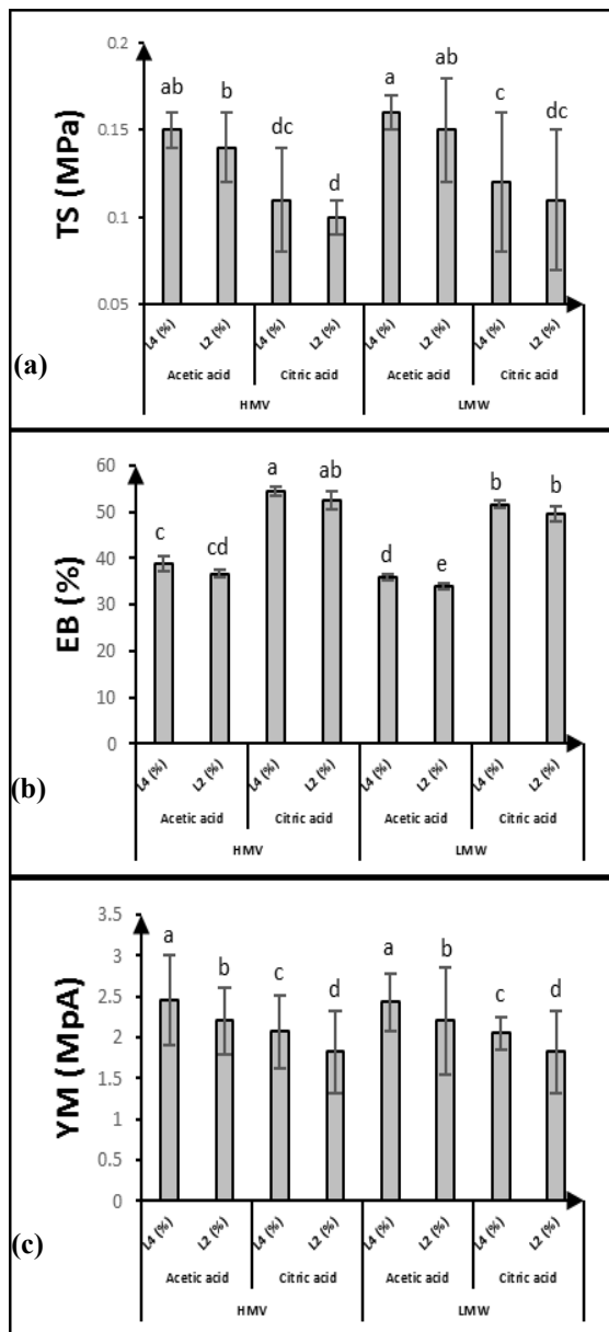
شکل (۲): اثرات متقابل سطح، وزن مولکولی و حلال بر استحکام کششی (TS) (a)، کشیدگی در نقطه شکست (EB) (b) و مدول یانگ (YM) (c) فیلم کیتوزان
