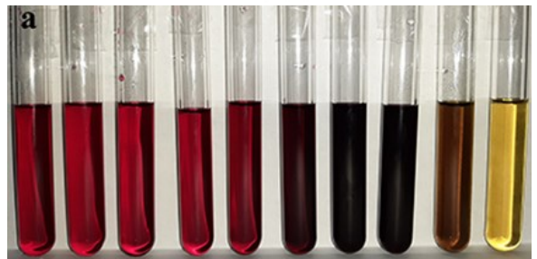
شکل (۷): پاسخ رنگی عصاره پوست ریشه چغندر قرمز در رنج pH ۳ تا ۱۲ (از چپ به راست) (شکل ۷a). مقادیر جذب نوری عصاره پوست ریشه چغندر قرمز تغییر رنگ یافته در طول موج ۳۰۰ تا ۸۰۰ نانومتر (شکل ۷b).
