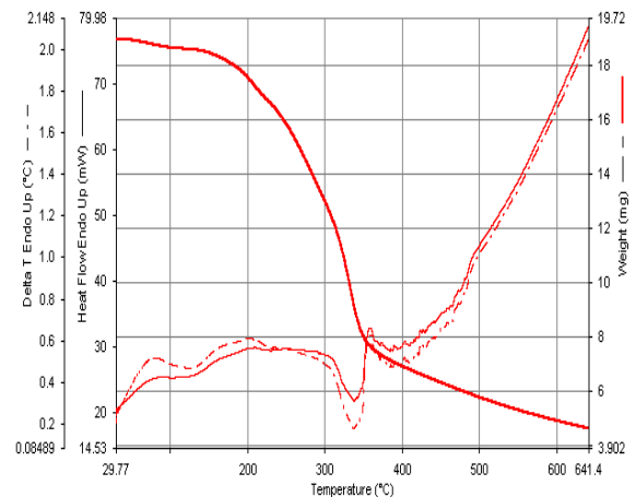
شکل (۵): منحنی کاهش وزن الیاف لیگنوسولوزی توسط دستگاه وزن سنج حرارتی
