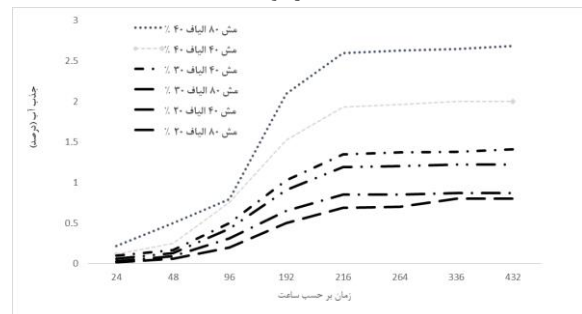
شکل (۴): منحنی جذب رطوبت در ۴۲°C ساعت قرارگیری در محفظه کليما تيزاسيون
